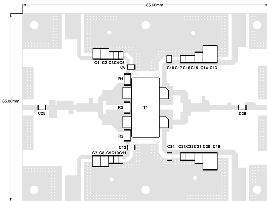
版图
