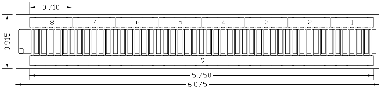
正视图
